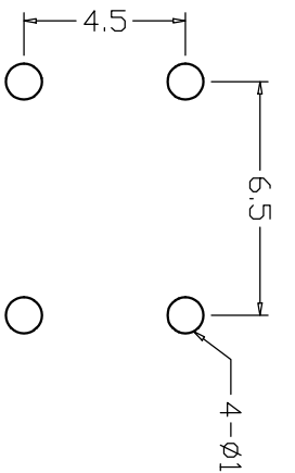
PCB线路板图
