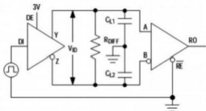
图6驱动时间测试电路
