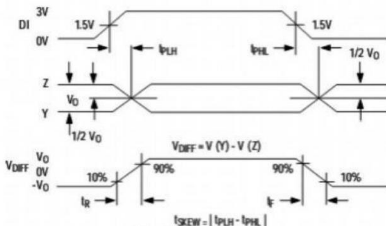
图 8 驱动传输延时
