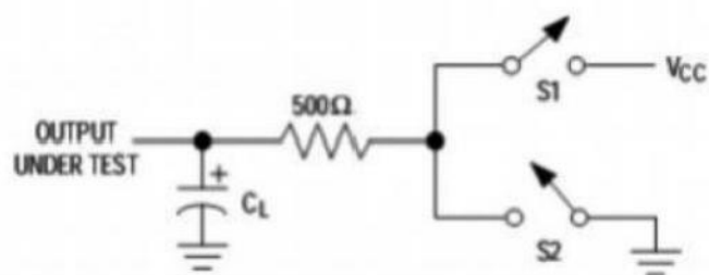
图6驱动时间测试电路
