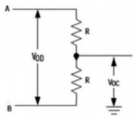
图3直流驱动测试电路
