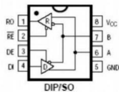
图1封装图
