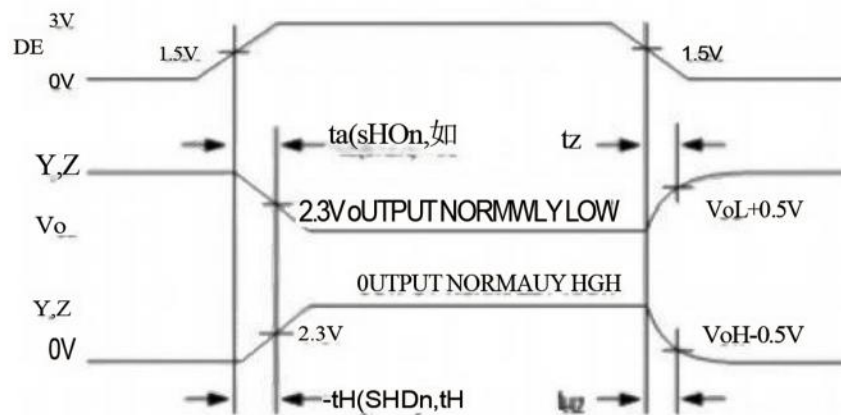
图10驱动开启和关闭时间
