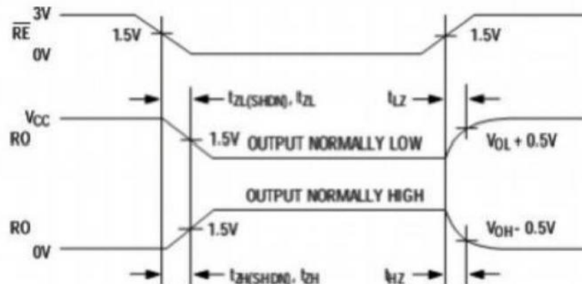
图 1 1 接收开启和关闭时间
