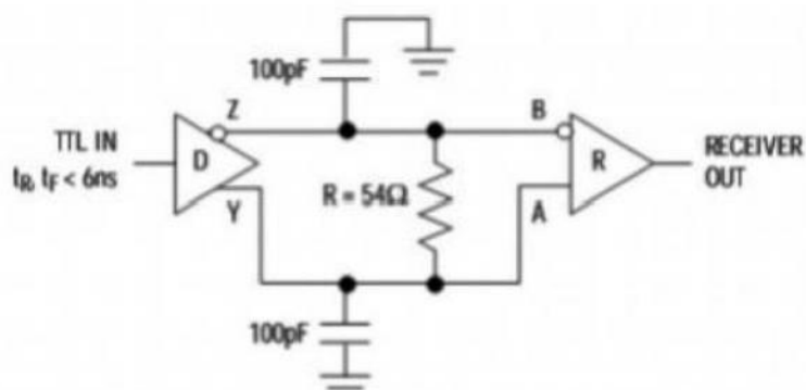
图7接收传输延时测试电路
