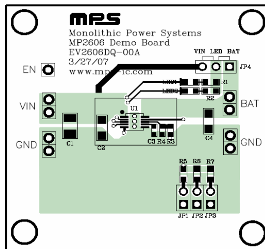
Figure 2—Top Layer
