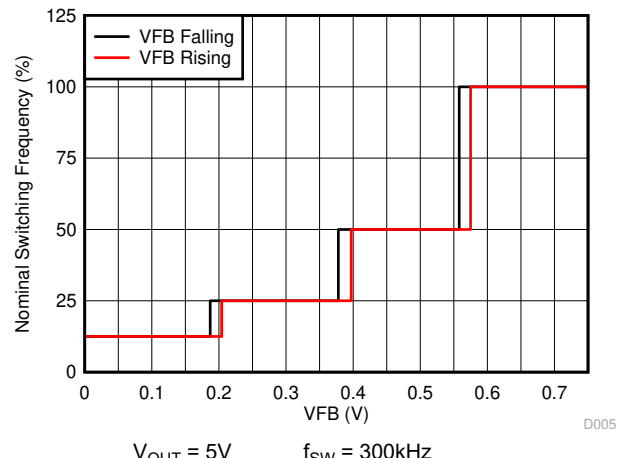
图 5-6. 频率与 V_{FB} 间的关系
