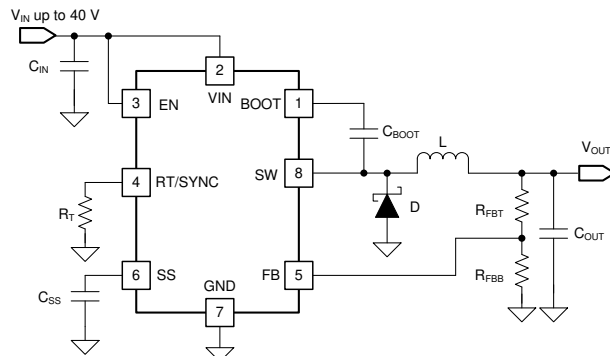
简化原理图
