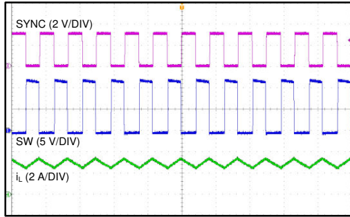
图 6-6. 在 CCM 下同步
