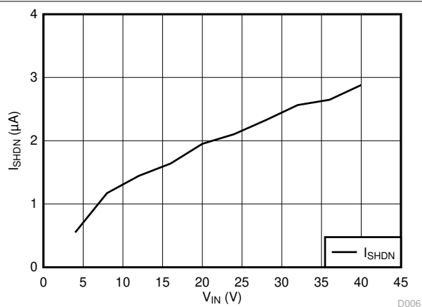
图 5-11. 关断电流
