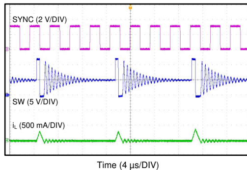
图 6-8. 在 PSM 下同步
