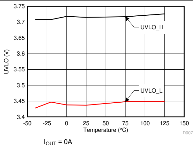
图 5-12. UVLO Threshold
