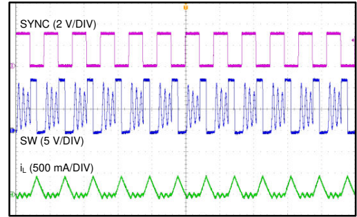
图 6-7. 在 DCM 下同步
