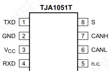
a. TJA1051T: SOP-8
