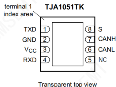
b. TJA1051TK: SOP-8
