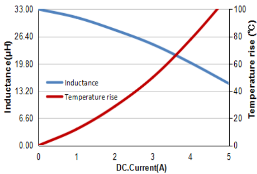
FSA0650-330MT
