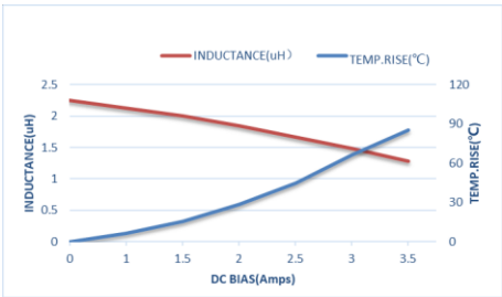
ZEPIM201608S-2R2M
