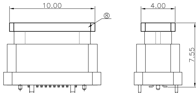
CAP尺寸图
