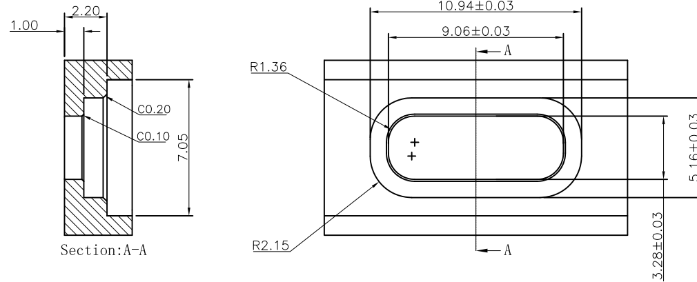
机壳开孔建议尺寸图
