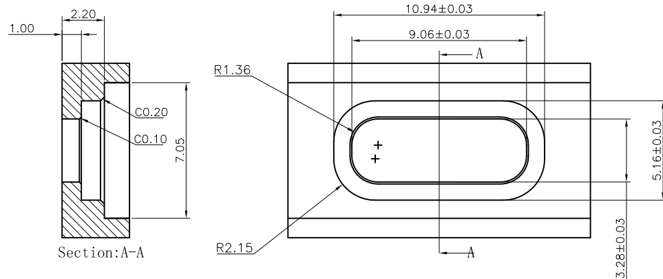
机壳开孔建议尺寸图 \triangle B
