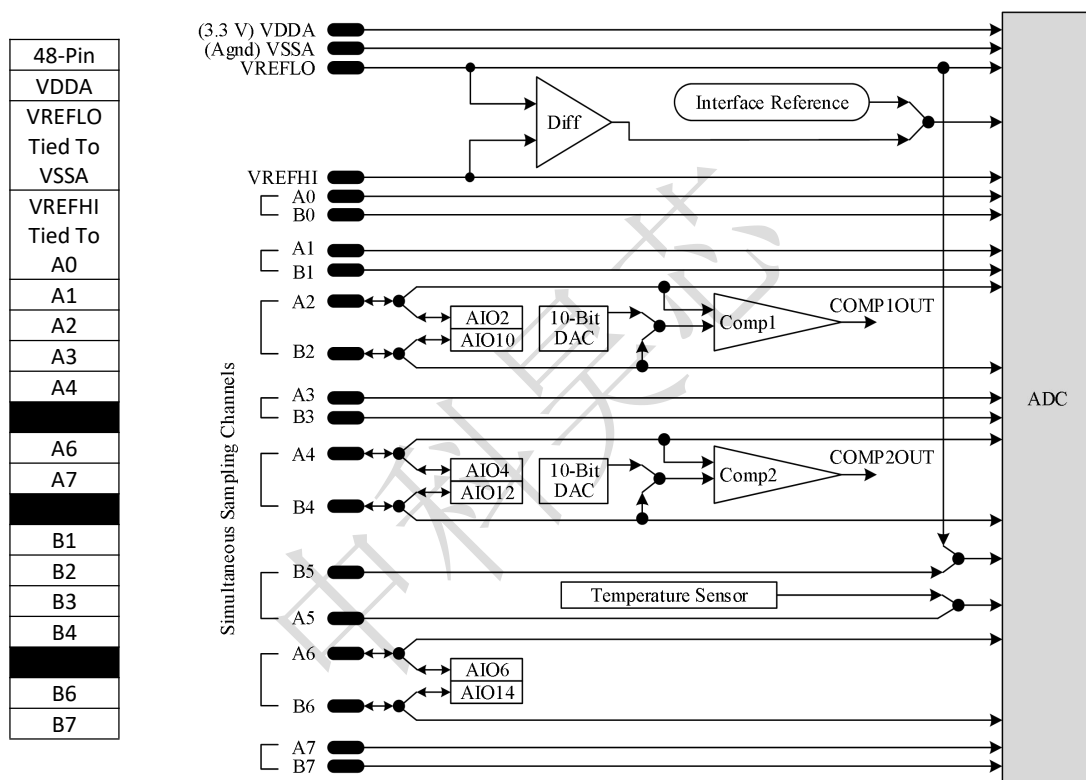
图 4-1 模拟引脚配置
