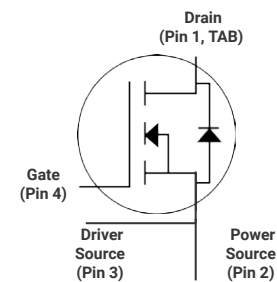
TO-247-4L Package
