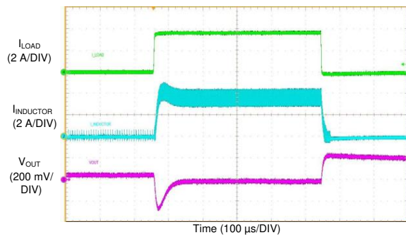
图 77. LM76003 Load Transient
