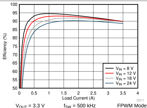
图 24. LM76003 Efficiency
