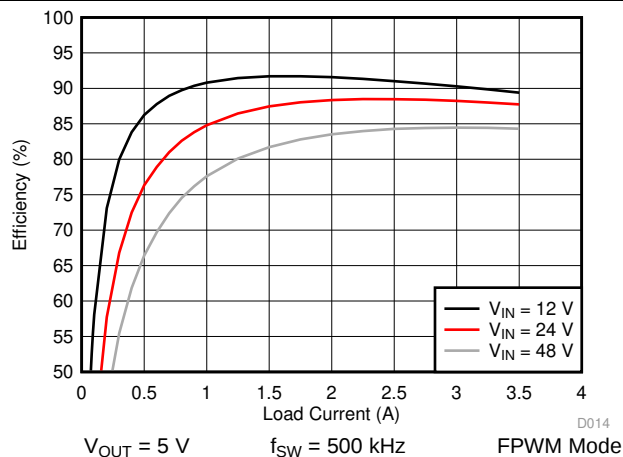
图 26. LM76003 Efficiency
