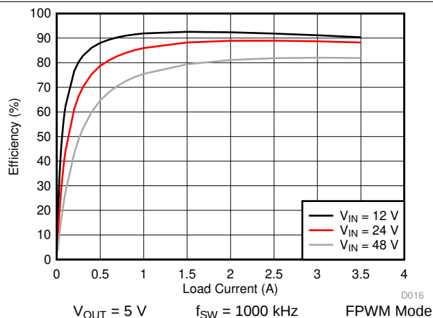
图 28. LM76003 Efficiency
