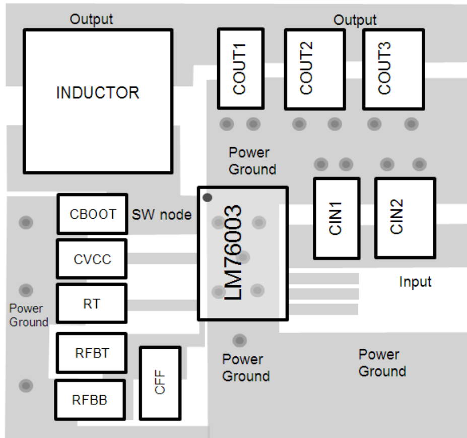
图 87. LM76002/LM76003 Layout
