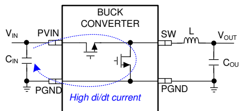
图 85. Buck Converter High di / dt Path
