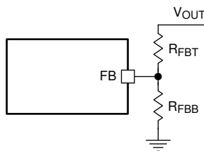
图 11. Output Voltage Setting
