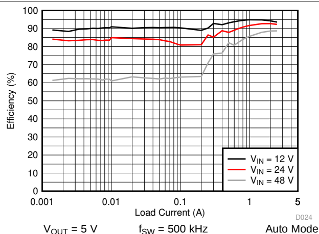
图 35. LM76002 Efficiency
