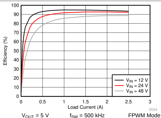
图 36. LM76002 Efficiency
