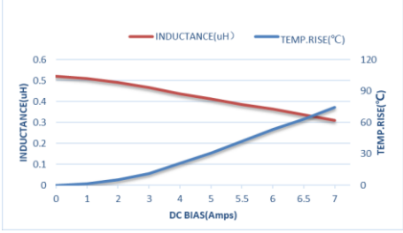
ZETC201608S-R47MT-LF
