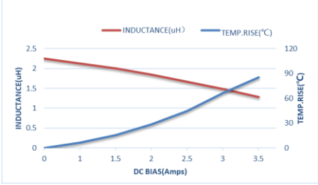
ZETC201608S-2R2MT-LF
