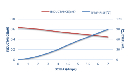
ZETC201608S-R68MT-LF
