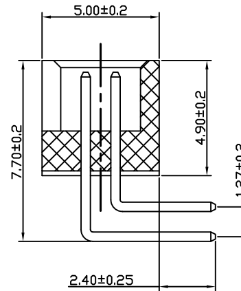
A-A SECTION
