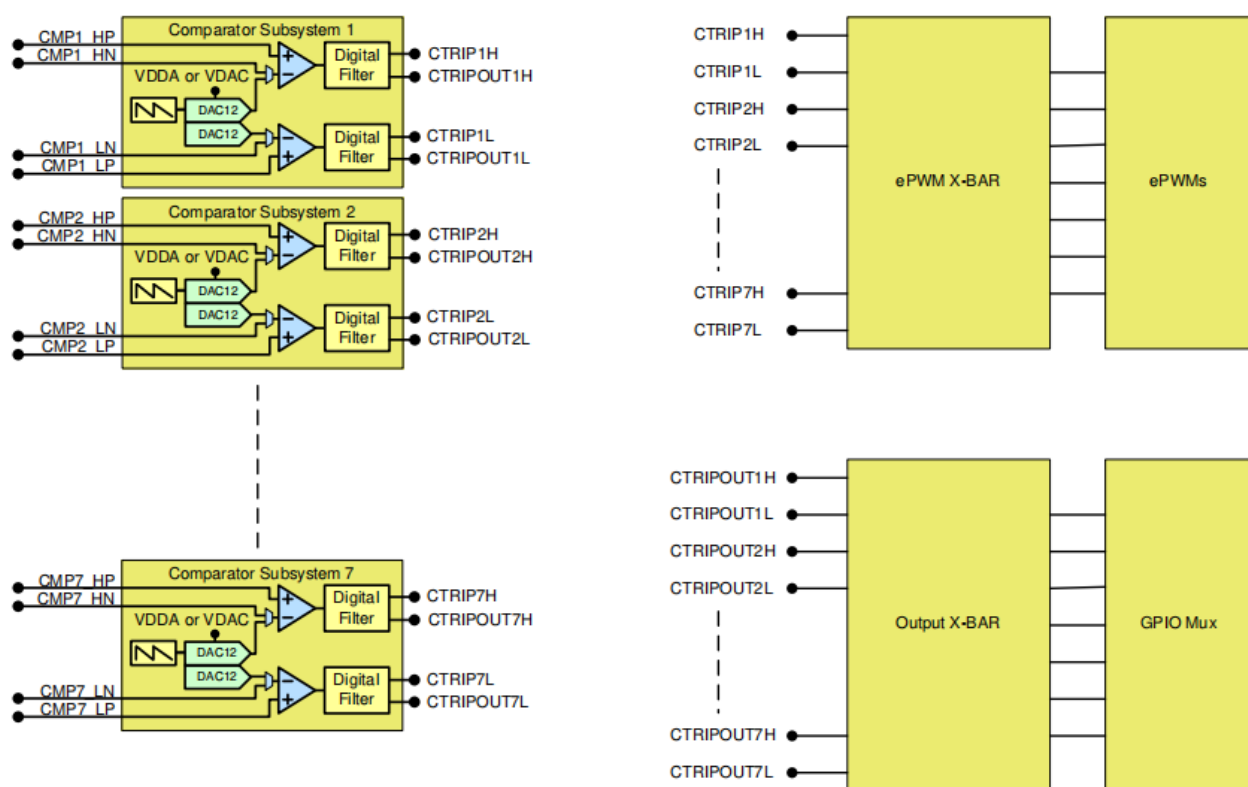
图 5-25 CMPSS 连接
