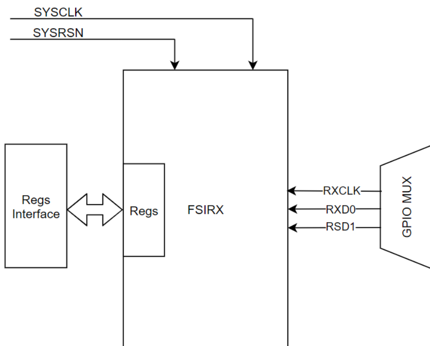
图 5-60. FSIRX CPU
