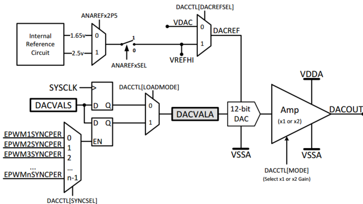
图 5-15. DAC 模块方框图
