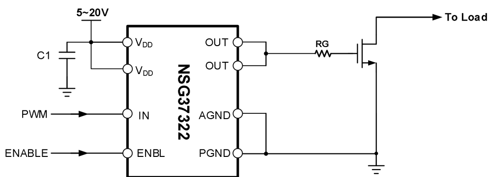
图 9-2 NSG37322 典型应用电路图
