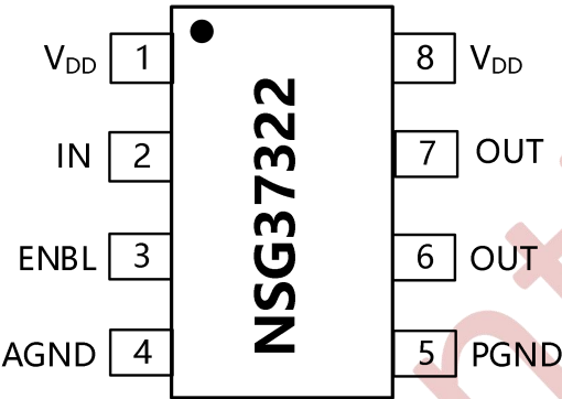
图 6-1 8 脚 SOP8 顶视图
