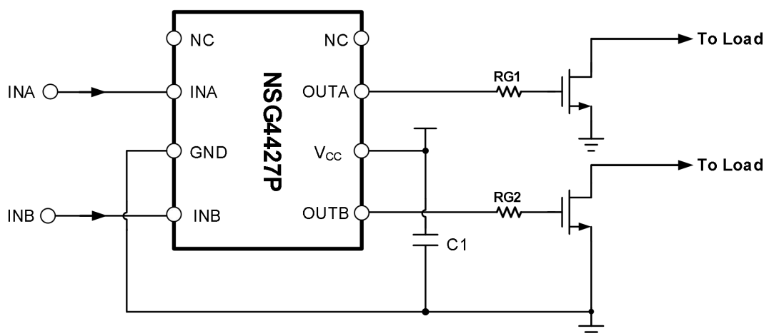
图 11-1 NSG4427P 典型应用电路图
