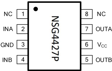
图 7-1 8-脚 DIP8 顶视图
