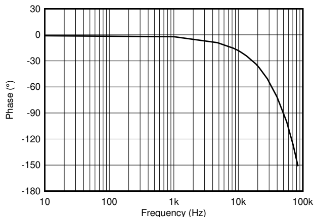
图 9-5. 归一化相位，所有型号
