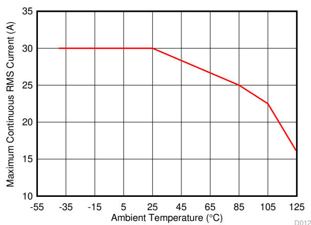
图 8-5. 最大连续 RMS 电流与环境温度间的关系
