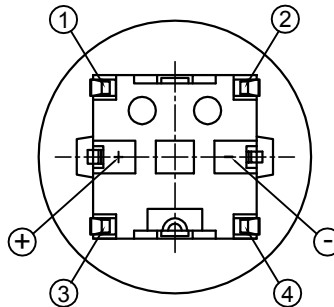
开关底部图
