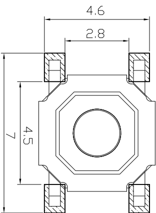
PCB 焊盘尺寸
