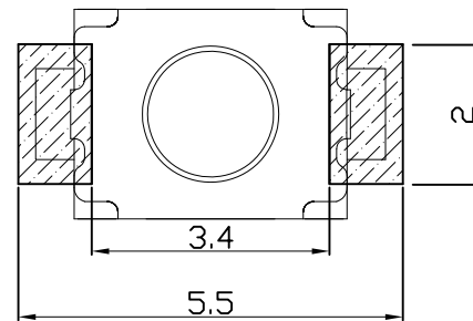
PCB 板焊盘尺寸
