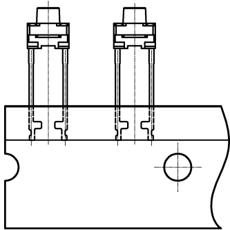
图1 编带图
