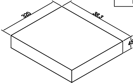
图3 内盒包装
