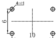
P. C. B. LAYOUT
