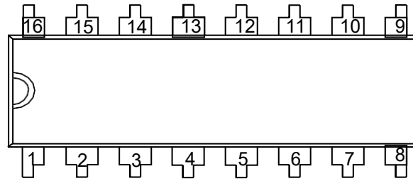
DIP-16/SOP-16/TSSOP-16/QSOP-16
