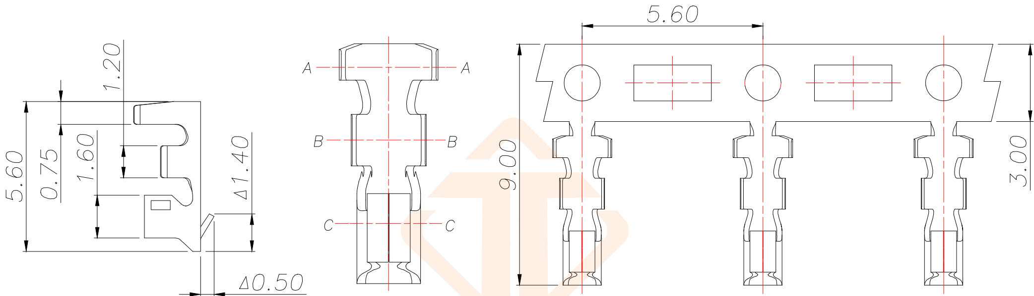
料带图 比例:1:2
