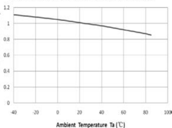
最大正向电流与环境温度特性曲线
