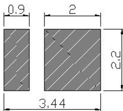
焊盘建议图
