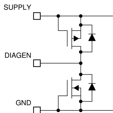
图 7-9. DIAGEN Pin
