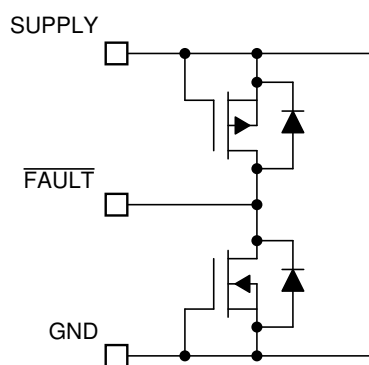
图 7-10. FAULT Pin
