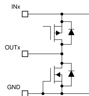
图 7-11. OUTx Pins
