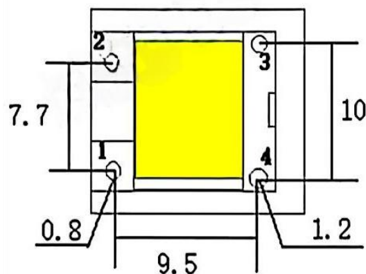
底视图
