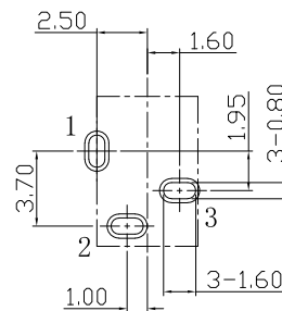
P. C. B 设计参考尺寸
