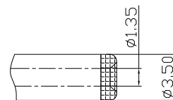
推荐插头尺寸
