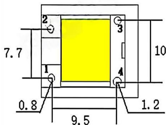
底视图
