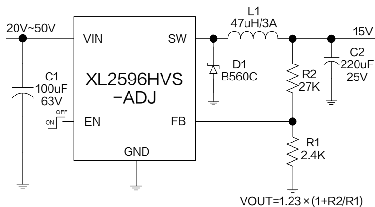
图 6. XL2596HVS-ADJ 系统参数测量电路 ( V_{OUT}=15V )
