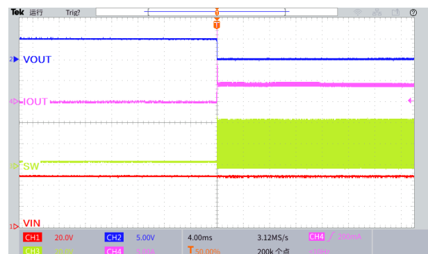
图 31.输出短路波形 ( V_{IN}=48V , V_{OUT}=5.0V )
