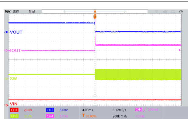
图 28.输出短路波形 ( V_{IN}=12V , V_{OUT}=5.0V )
