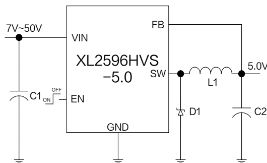
图1.XL2596HVS-5.0典型应用示意图和转换效率曲线
