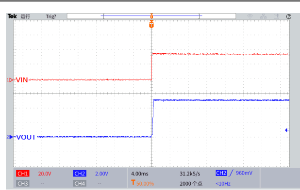
图 26.上电波形图 ( V_{IN}=36V , V_{OUT}=5.0V , I_{OUT}=0.1A )
