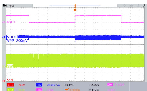
图 34.瞬态负载响应波形 ( V_{IN}=36V , V_{OUT}=5.0V , I_{OUT}=0.1 至 2A )
