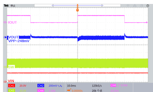
图 33.瞬态负载响应波形 ( V_{IN}=24V , V_{OUT}=5.0V , I_{OUT}=0.1 至 2A )
