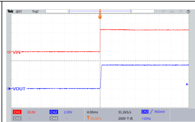
图 25.上电波形图 ( V_{IN}=24V , V_{OUT}=5.0V , I_{OUT}=0.1A )
