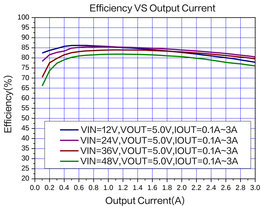
图 5. XL2596HVS -ADJ 系统效率曲线
