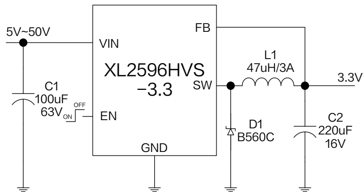
图 8.XL2596HVS-3.3 系统参数测量电路
