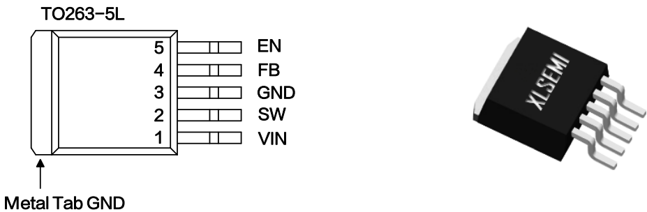
图 2. XL2596HVS 引脚配置
