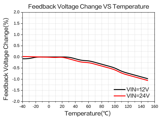
图 18.反馈电压温度系数曲线图
