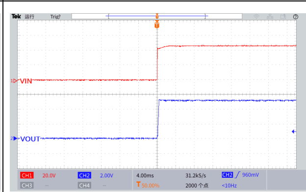
图 27.上电波形图 ( V_{IN}=48V , V_{OUT}=5.0V , I_{OUT}=0.1A )
