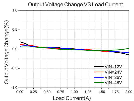
图 15.负载调整率曲线图
