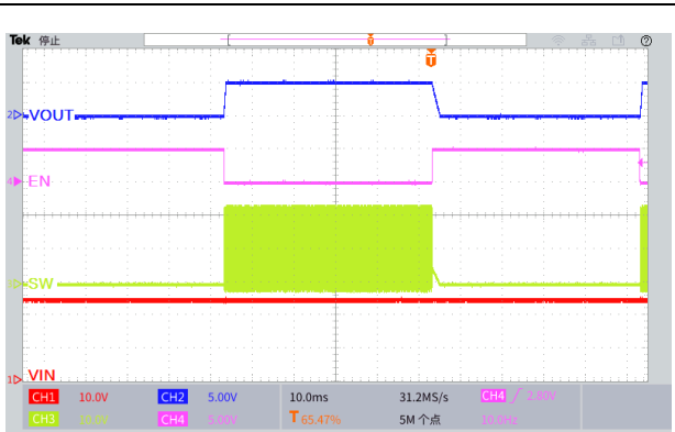
图 37.EN 引脚开关机波形 ( V_{IN}=24V , V_{OUT}=5.0V , I_{OUT}=0.5A )
