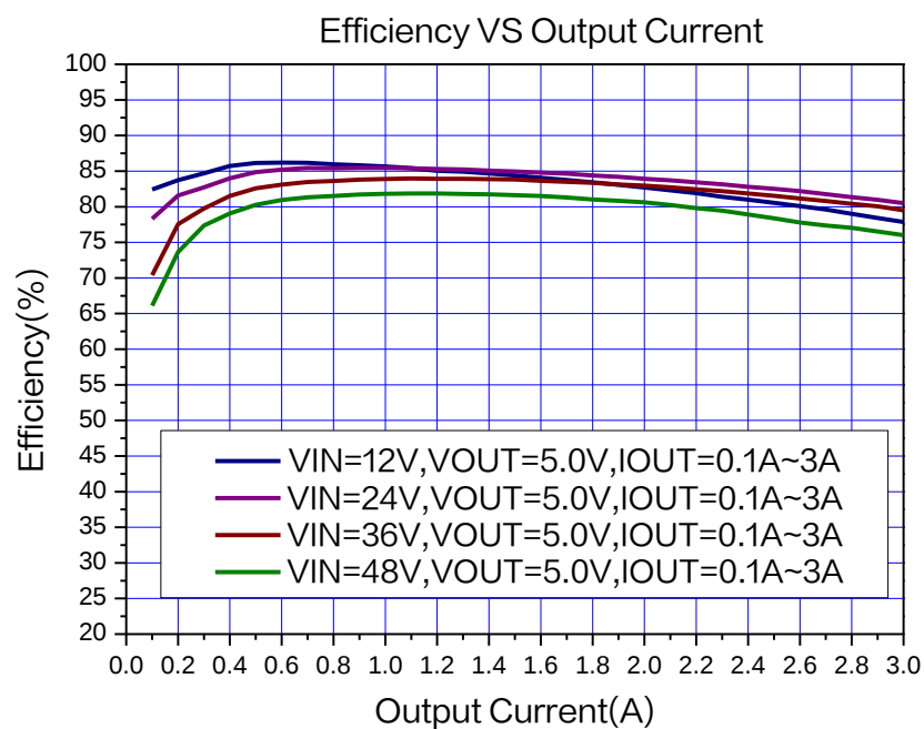
图 11. XL2596HVS-5.0 系统效率曲线
