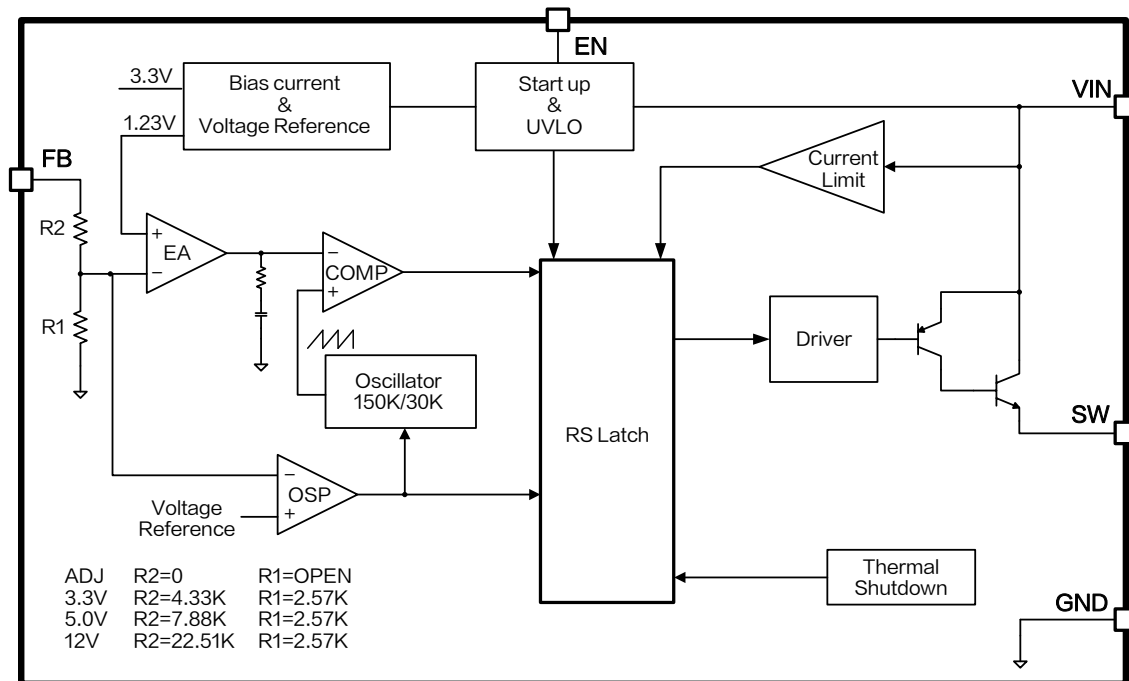
图 3. XL2596HVS 方框图
