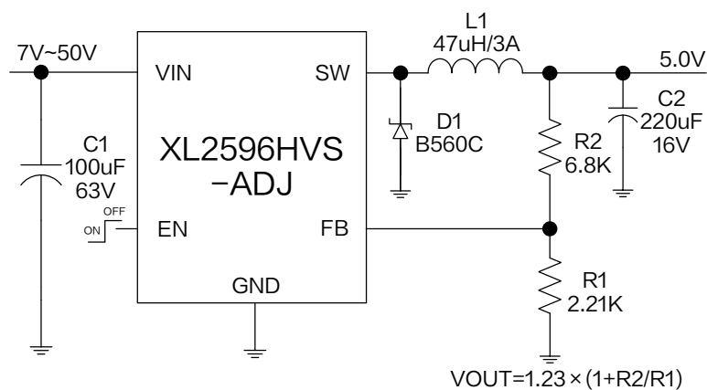
图 4 XL2596HVS-ADJ 系统参数测量电路 ( V_{OUT}=5.0V )
