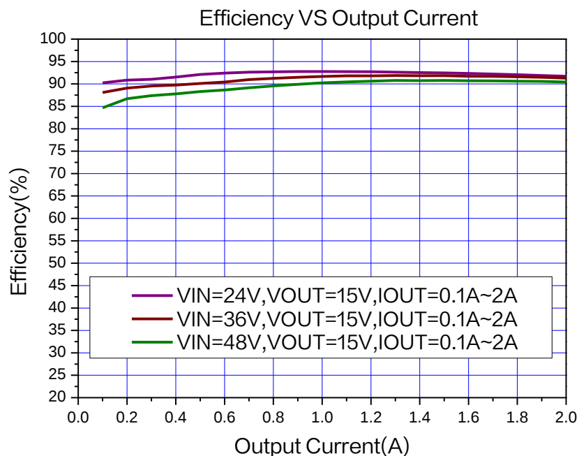
图 7. XL2596HVS-ADJ 系统效率曲线
