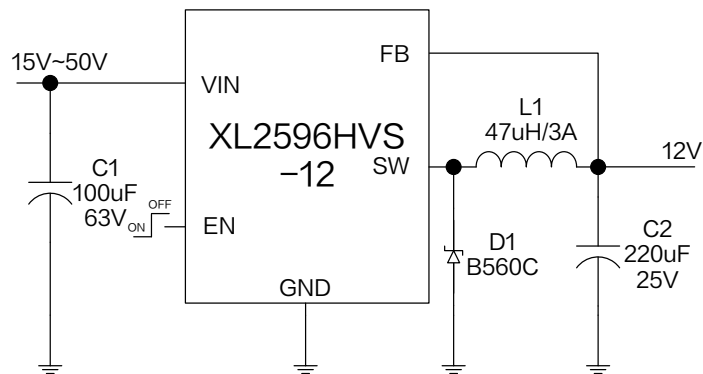
图 12.XL2596HVS-12 系统参数测量电路
