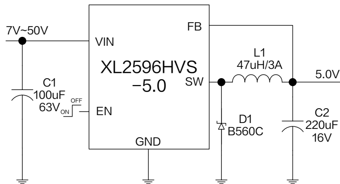
图 10.XL2596HVS-5.0 系统参数测量电路
