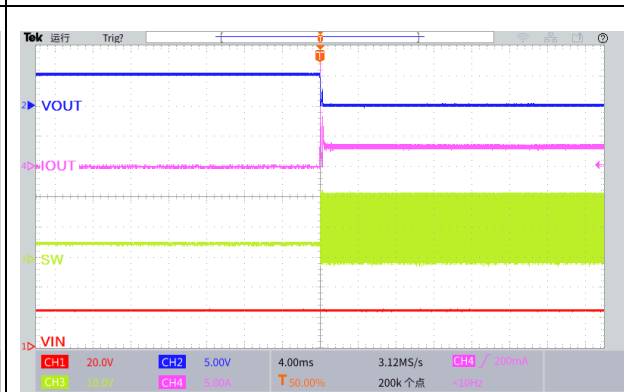
图 29.输出短路波形 ( V_{IN}=24V , V_{OUT}=5.0V )
