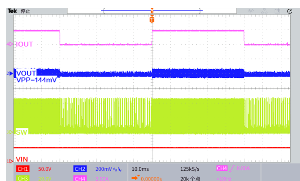
图 35.瞬态负载响应波形 ( V_{IN}=48V , V_{OUT}=5.0V , I_{OUT}=0.1 至 2A )
