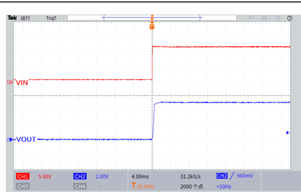
图 24.上电波形图 ( V_{IN}=12V , V_{OUT}=5.0V , I_{OUT}=0.1A )
