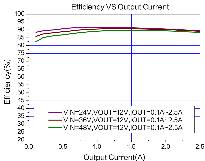
图 13. XL2596HVS-12 系统效率曲线
