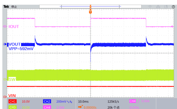
图 32.瞬态负载响应波形 ( V_{IN}=12V , V_{OUT}=5.0V , I_{OUT}=0.1 至 2A )
