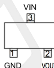
SOT23-3L & SOT23
