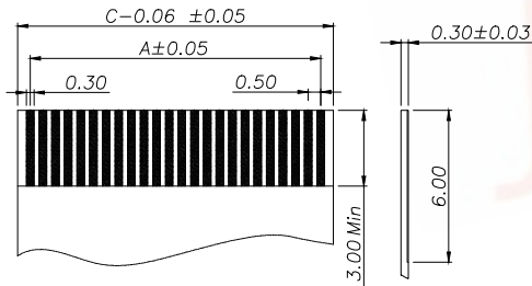
通用FFC寸法 Applicable FFC
