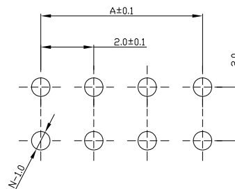
PCB参考图
