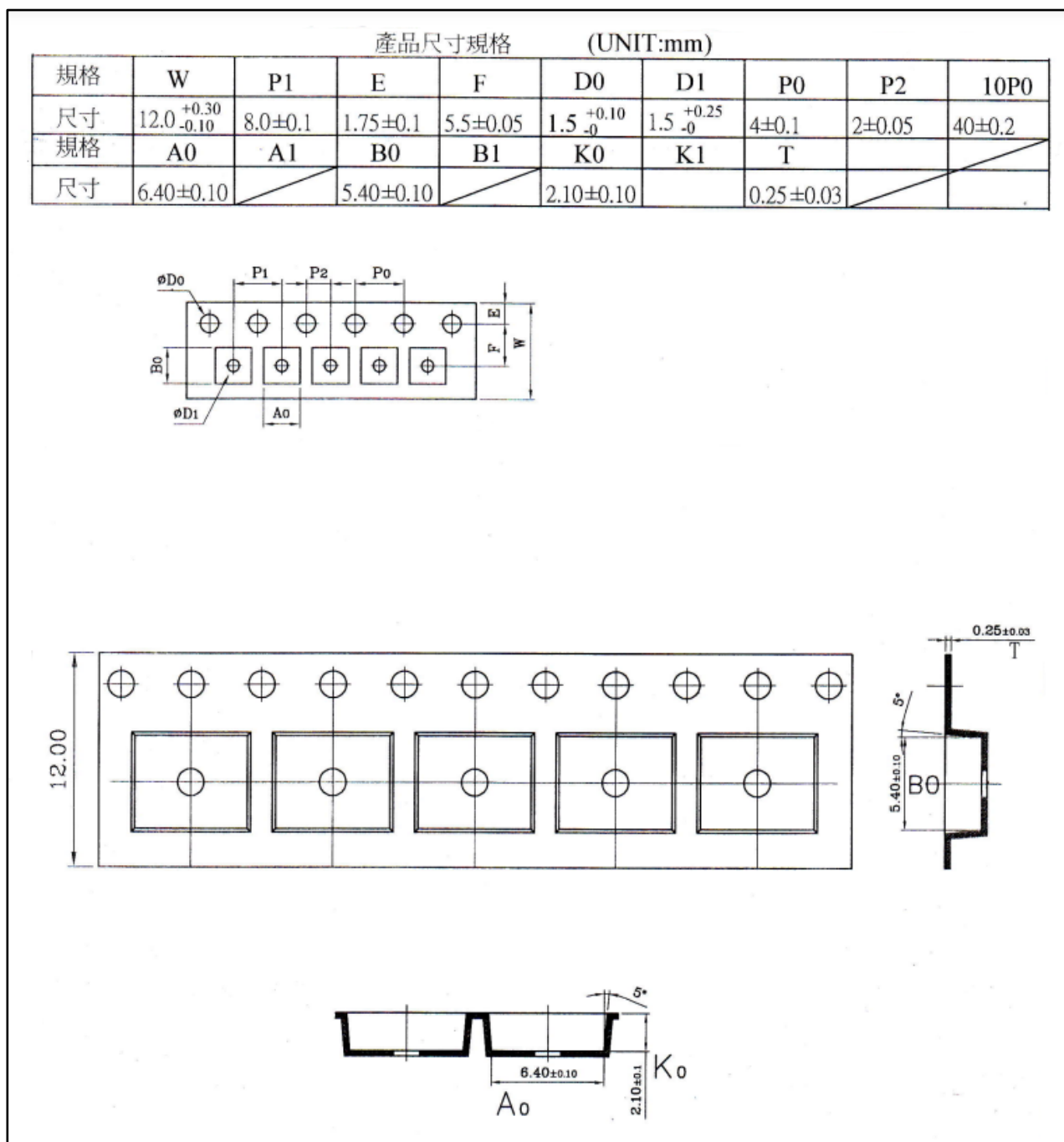
图 26.CMT812X NB SOIC-8 编带信息
