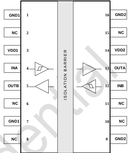
图 3. CMT8122WXM 管脚
