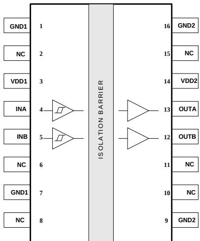
图 1. CMT8120WXM 管脚
