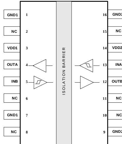
图 2. CMT8121WXM 管脚
