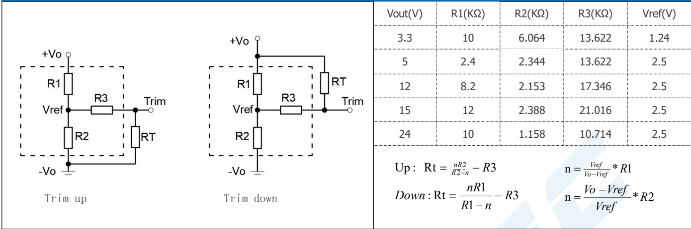
应用电路（图 4）
