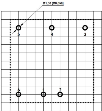
栅格距离尺寸为 2.54 x 2.54 mm
