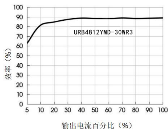
效率 VS 输出负载曲线图（ V_{in}=48V ）
