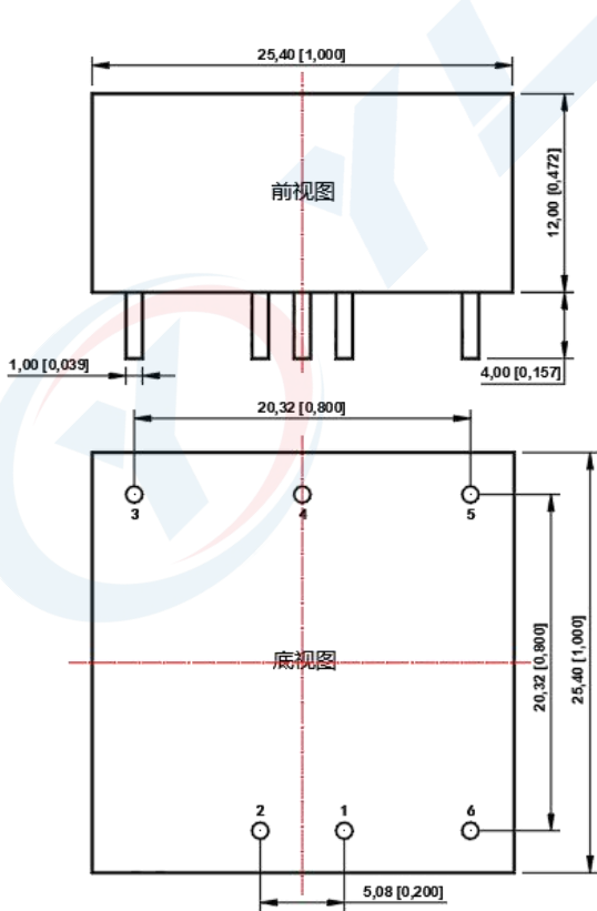
外观尺寸图
