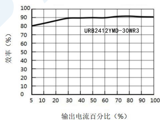
效率 VS 输出负载曲线图（ V_{in}=48V ）
