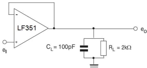
电压跟随器
