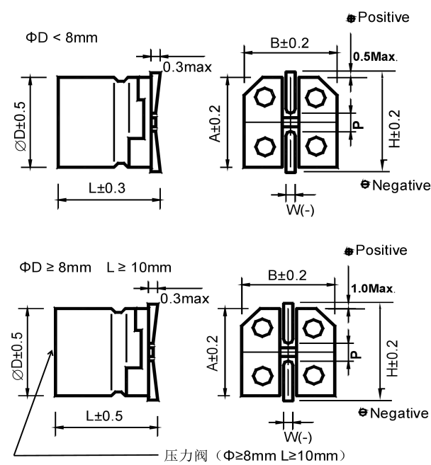
标准尺寸图：
