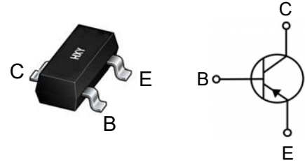
SOT-23
