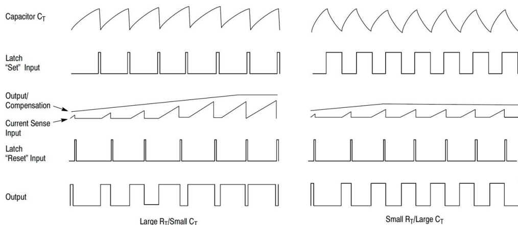
时序图
