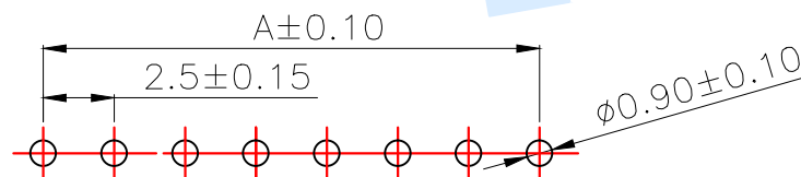
适用线路板 (PCB LAYOUT)
