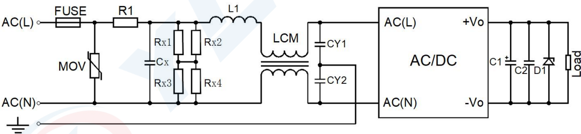
EMC 解决方案-推荐电路（图 2）
