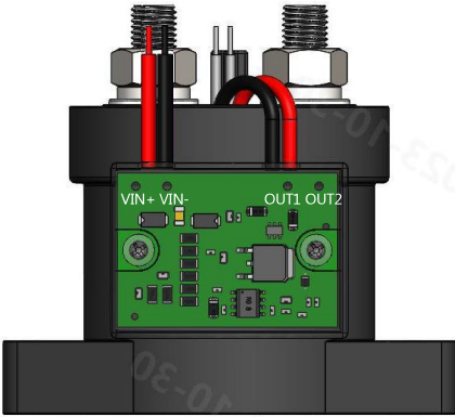
图 2 搭配接触器应用图
