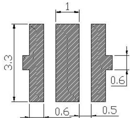
焊盘建议图
