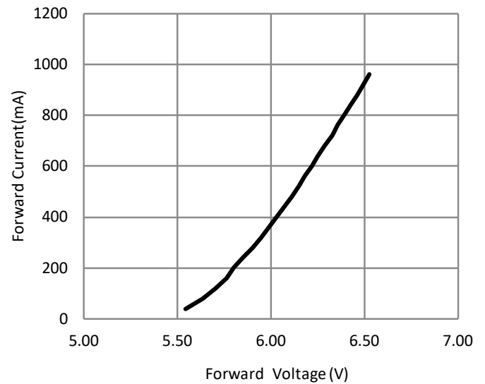
V_f ----- I_f
