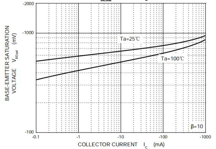
V_{BEsat} — I_c
