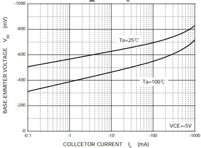
V_{BE} — I_c
