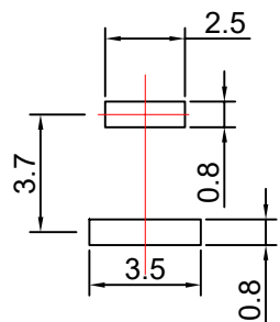
PCB 开孔尺寸
