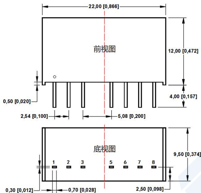
外观尺寸图
